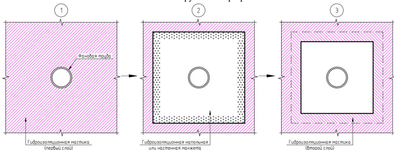
Рис.14.4. Последовательность нанесения гидроизоляционной манжеты
